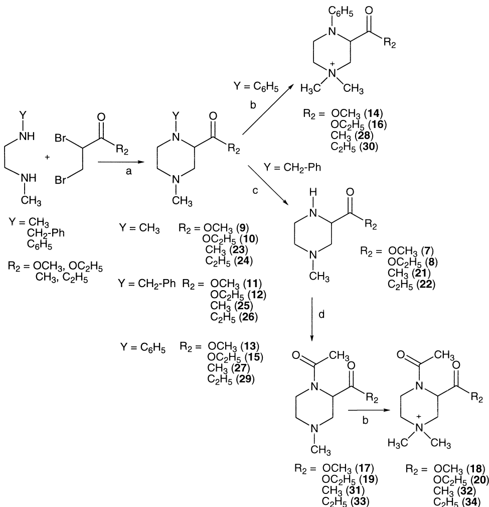
Scheme 1. (a) Anhyd. benzene/ \text{N}(\text{C}_2\text{H}_5)_3 ; (b) \text{CH}_3\text{I} ; (c) \text{Pd/C}/\text{H}_2 ; (d) \text{CH}_3\text{COCl} .
