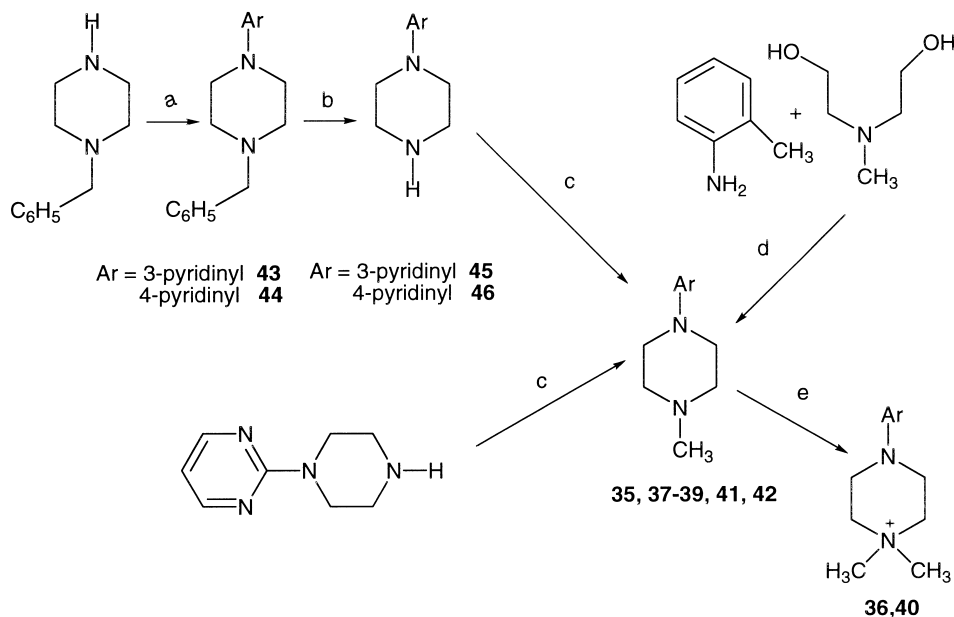
Scheme 2. (a) 3- or 4-bromopyridine; (b) Pd/C/H 2 ; (c) CH 2 O/HCOOH; (d) HCl, high temp. (e) CH 3 I.
